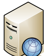
LINUX
